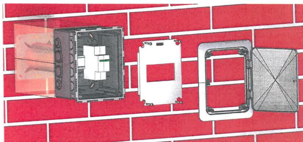
Použití jako úplný kryt dle ČSN EN 60670-24
