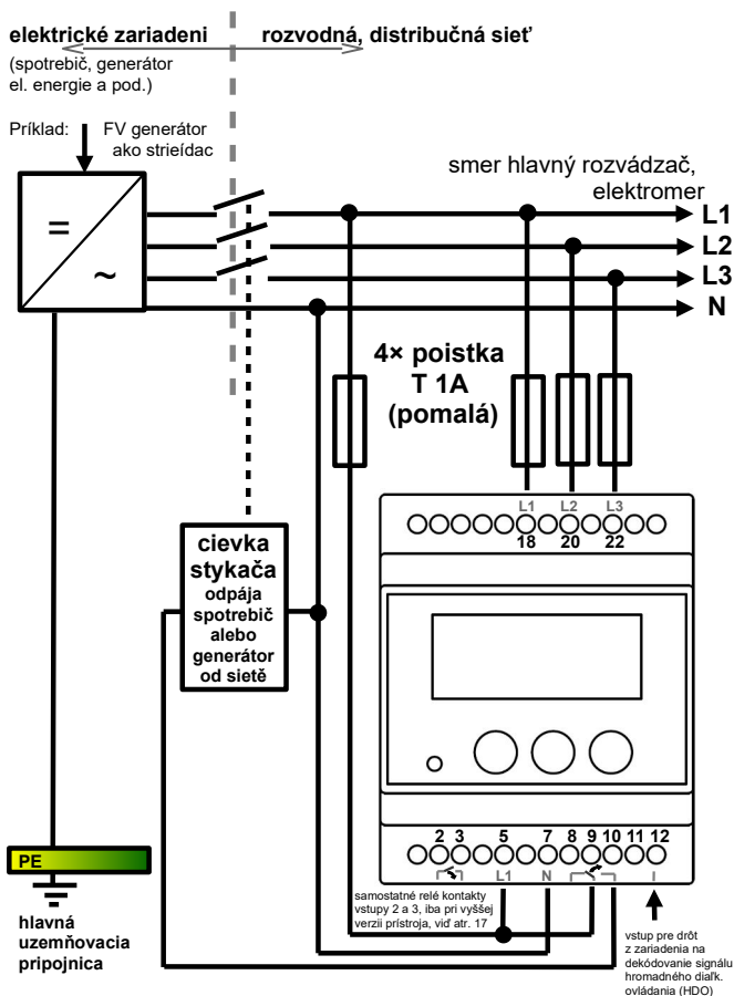
Obr. 1: Schéma zapojenia zariadenia
